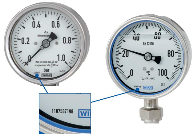
Манометры и показывающие термометры
